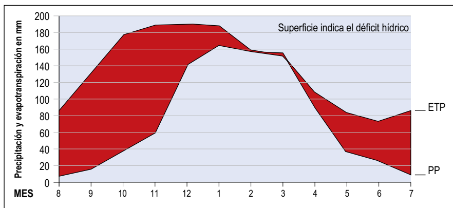
Figura 18: Precipitación (pp) y evapotranspiración (ETP) medias en el periodo 1978-1995V VVFuente: CIPCA y SNV 1996.
