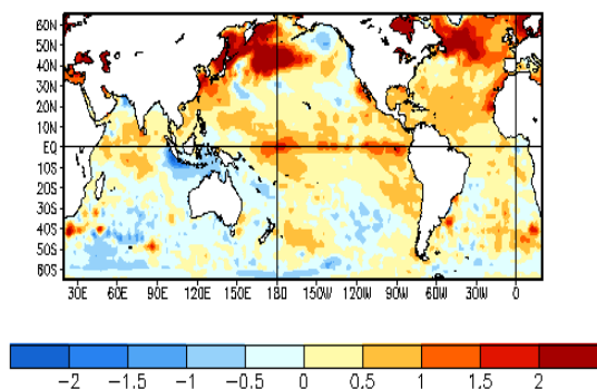
Figura 2. Temperatura Superficial del Mar global entre el 20 de agosto 16 de septiembre del 2006. (Fuente: NOA, 2006)
