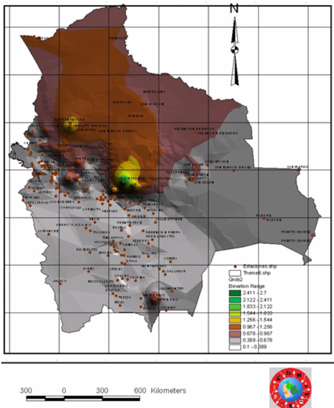
Mapa 8. Índices de aridez para Bolivia bajo condiciones de escenario de elevación de 1.5 °C de temperatura e incremento de 15 % de precipitación para los llanos y reducción del 15 % de precipitación para valles y altiplano. (Cuanto más bajo el valor, mayor es la aridez presentada por la zona evaluada)
