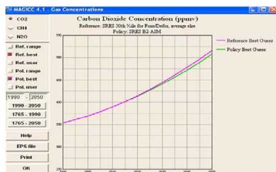
Figura 6. Incremento de las concentraciones atmosféricas de CO 2 bajo los supuestos del escenario B2-AIM.
